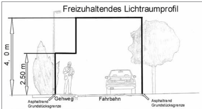
Lichtraumprofil: Das Lichtraumprofil zeigt, wie viel Raum zur Straße hin frei bleiben muss.
